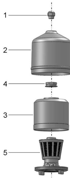
Рисунок 20 – Очистка ротора центробежного масляного фильтра
