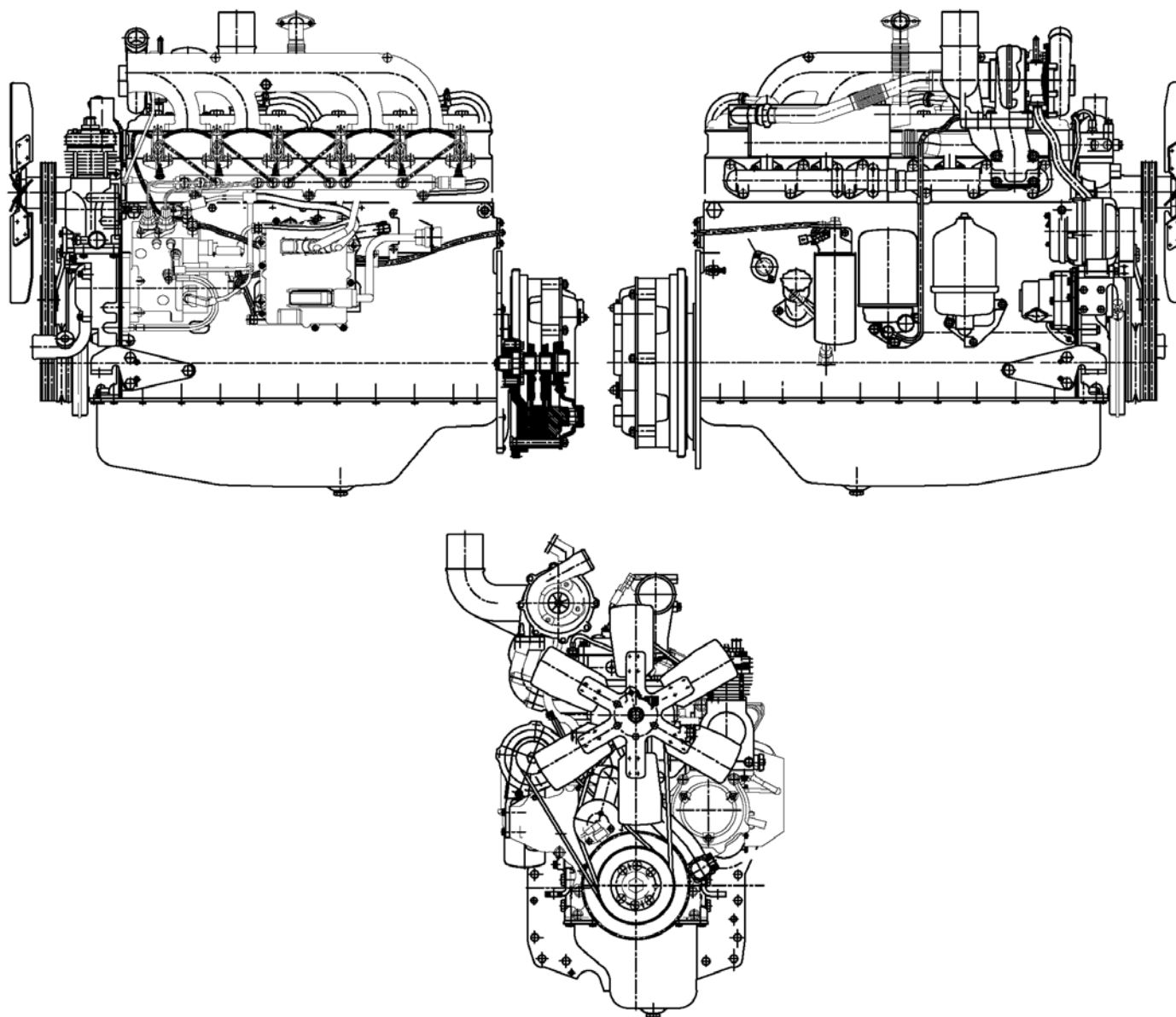
Рисунок 1 – Дизель Д-260.1S3A
