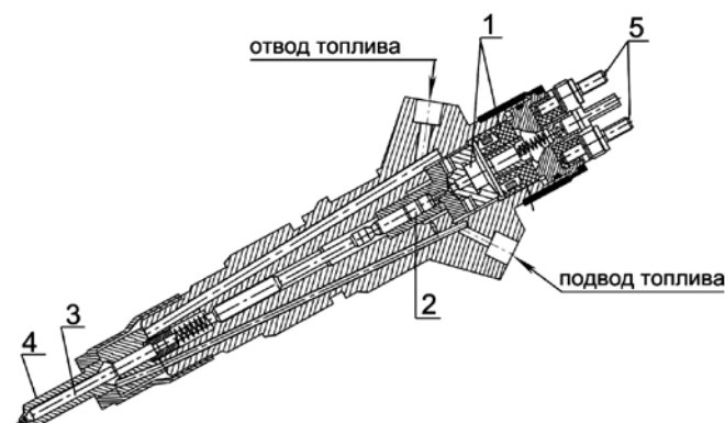
1 – электромагнитный клапан; 2 – управляющий клапан; 3 – игла распылителя; 4 – корпус распылителя; 5 – клеммы.
