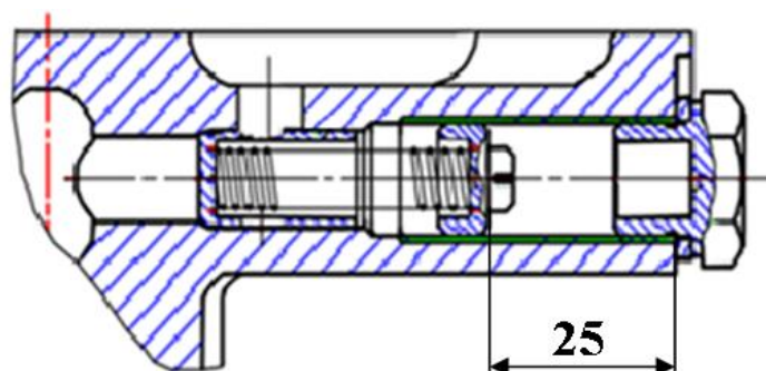
Рисунок 3.9 – Максимально допускаемый размер.
