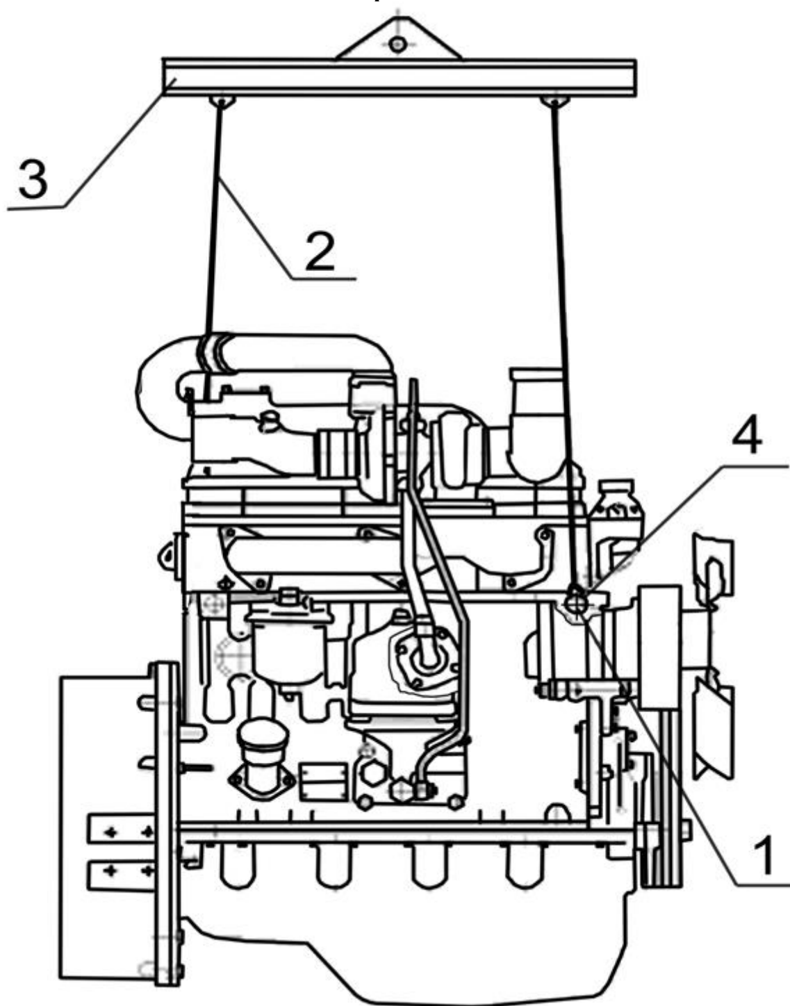
Рисунок Ж.1 – Схема строповки двигателя.
