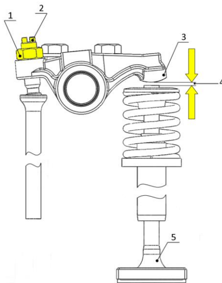
1 – контргайка; 2 – винт регулировочный; 3 – боек коромысла; 4 – зазор; 5 – клапан.
