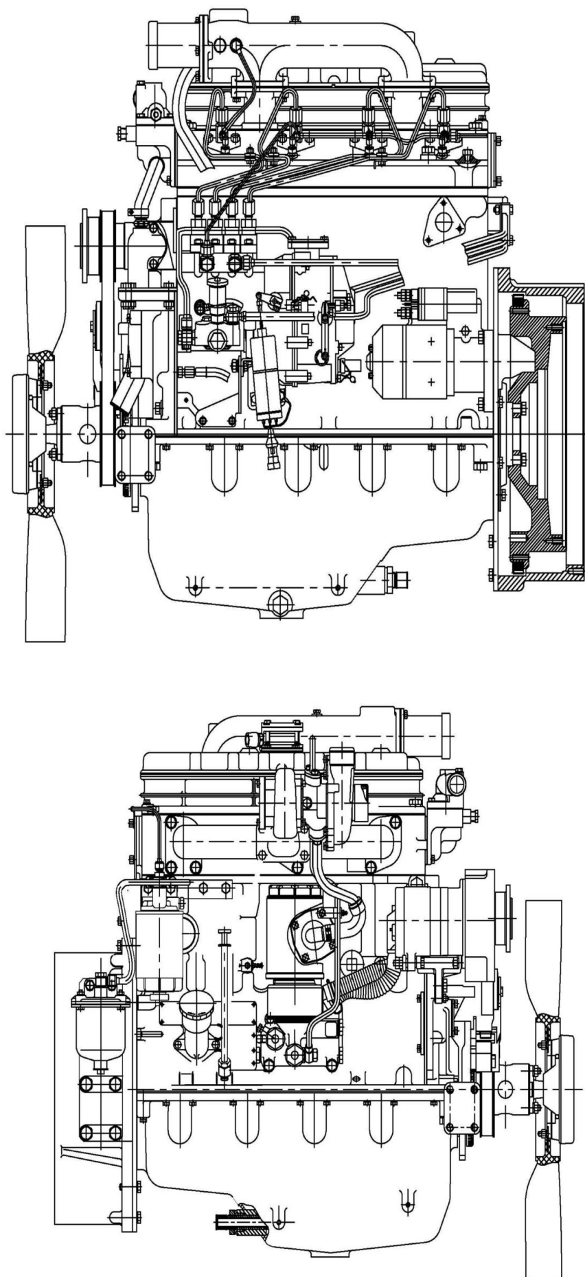
Рисунок 1.4 – Общий вид двигателя Д-246.10, Д-246.11.
