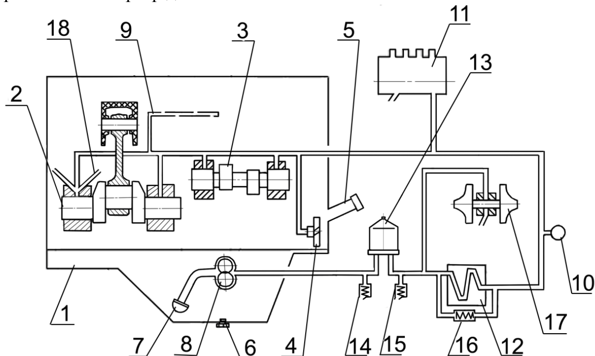
Рисунок 1.7 – Схема системы смазки двигателей Д-246.2, Д-246.3, Д-246.4, Д-246.7, Д-246.8, Д-246.9, Д-246.10, Д-246.11
