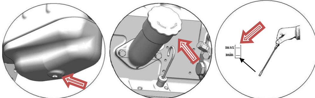
Рисунок 19 – Порядок замены масла в картере дизеля
