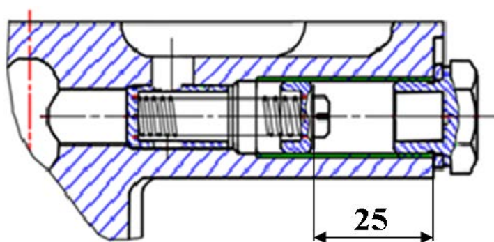
Рисунок 22 – Максимально допускаемый размер
