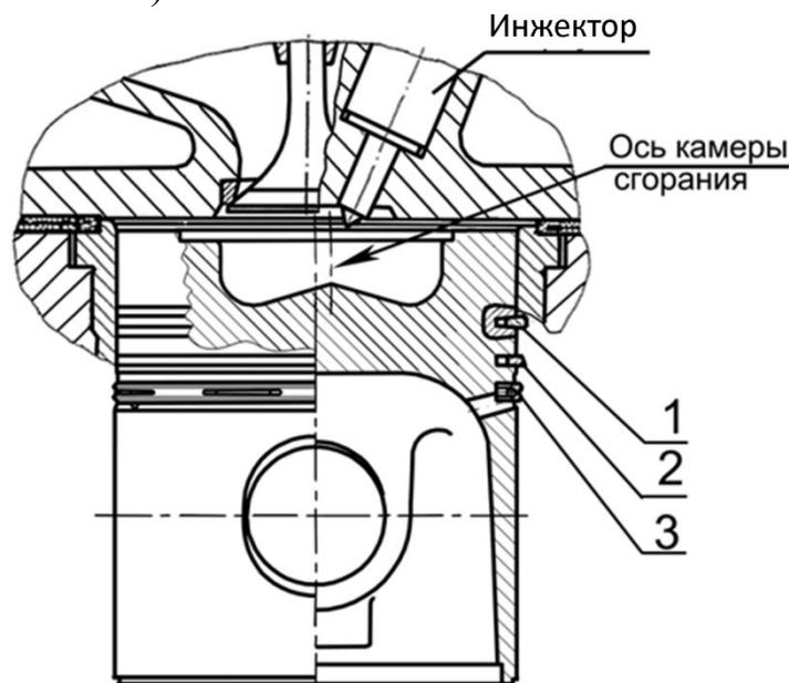
Рисунок 28 – Схема установки поршневых колец.
