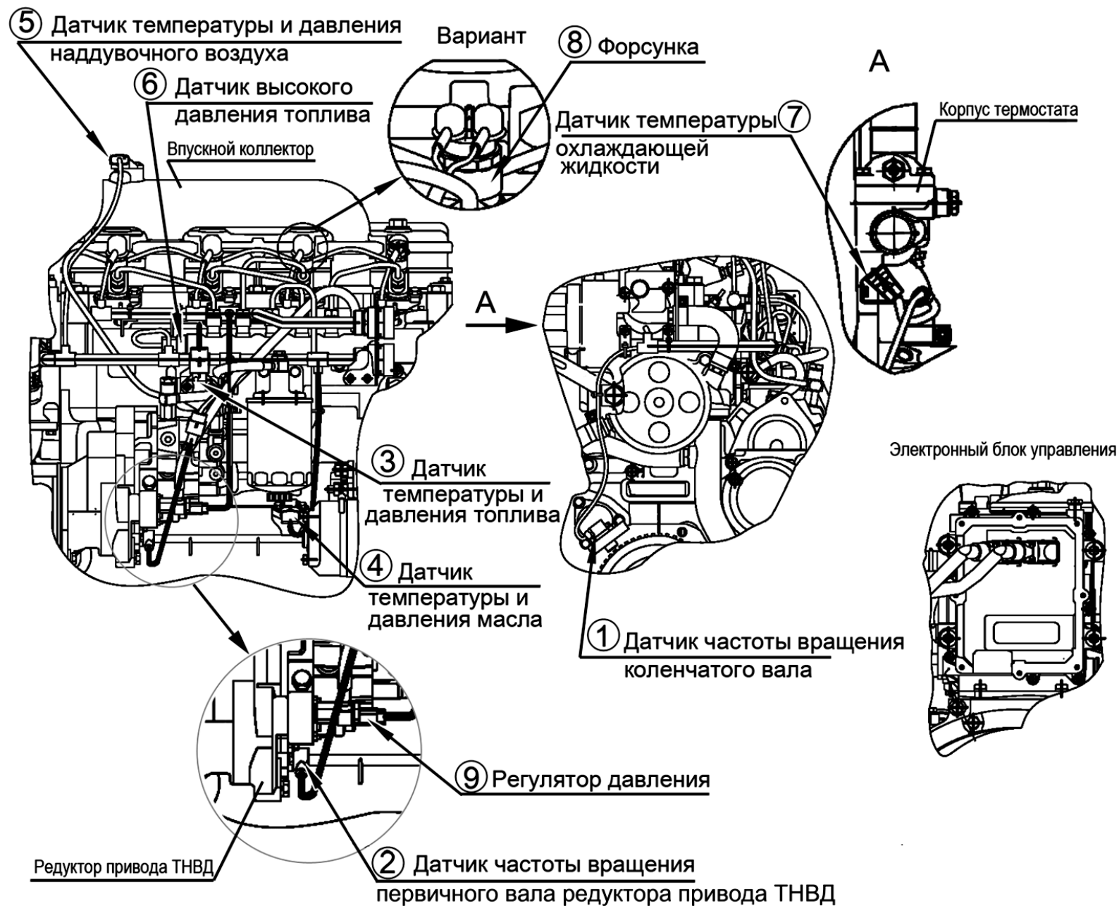
Рисунок 4 – Расположение датчиков и исполнительных механизмов.
