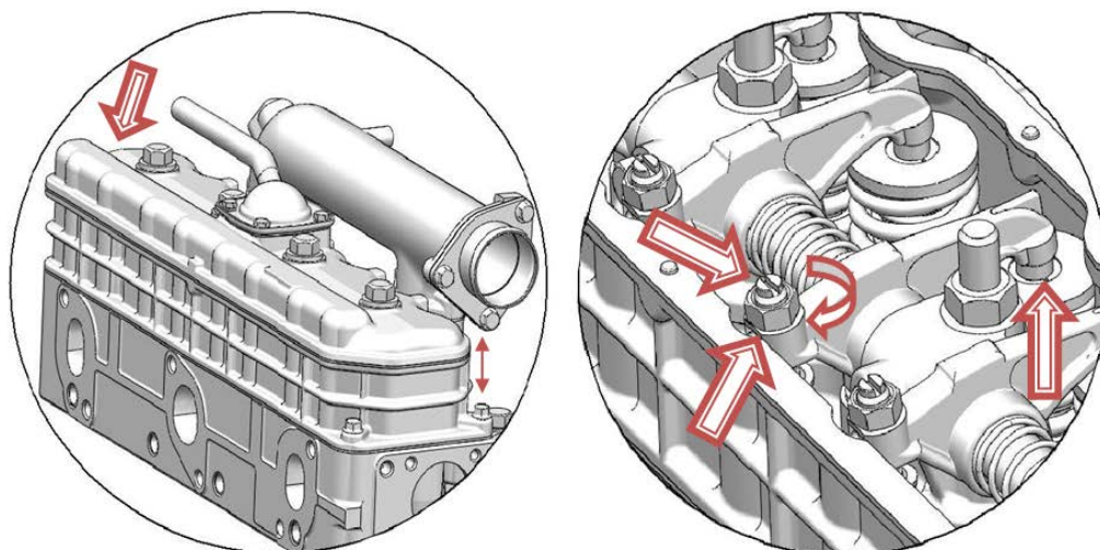
Рисунок 26 – Регулировка зазора в клапанах
