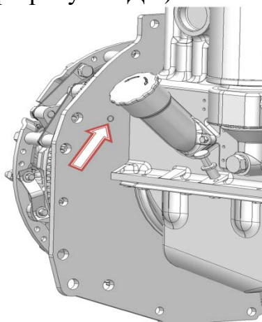
Рисунок Д.2 – Место установки фиксатора в отверстие заднего листа.
