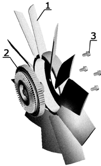
Рисунок 14 – Вентилятор с вязкостной муфтой отключения.
