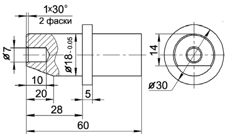
Рисунок Д.1 – Приспособление для фиксации установочного штифта.
