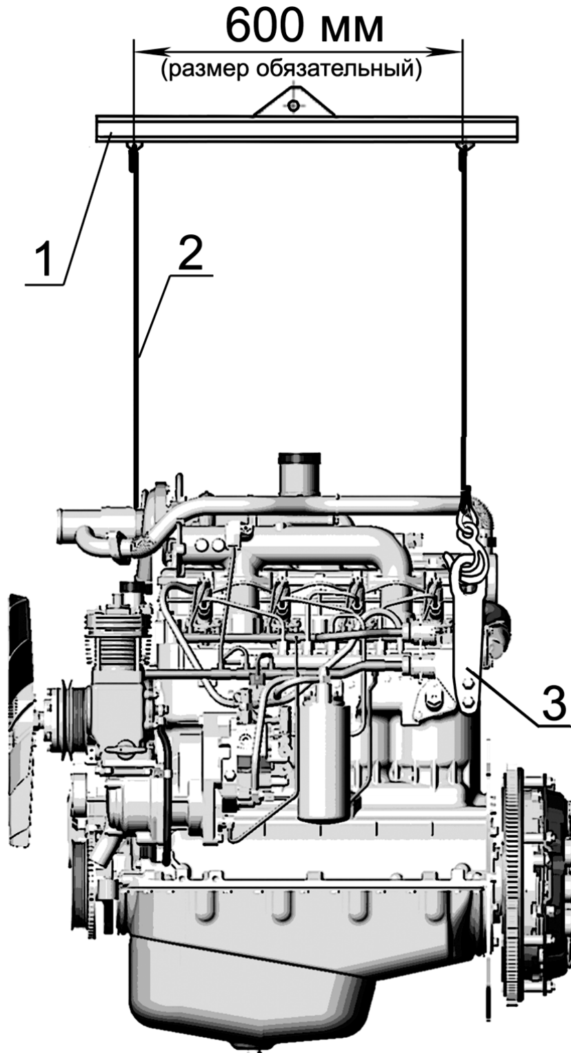
Рисунок К.1 – Схема строповки дизеля.
