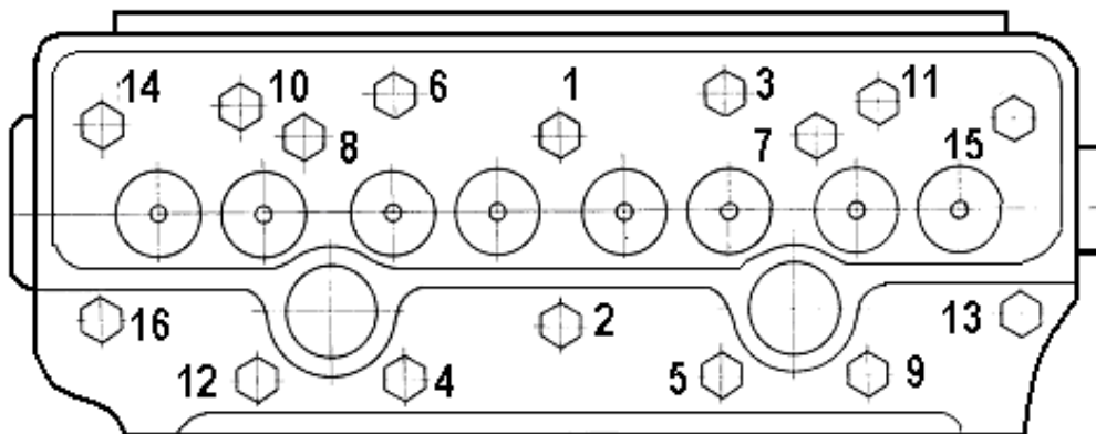
Рисунок 32 – Схема последовательности затяжки болтов крепления головки цилиндров
