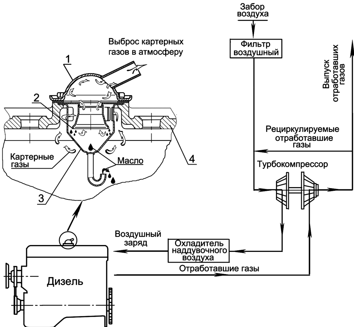
Рисунок – 13 Схема газообмена дизеля.
