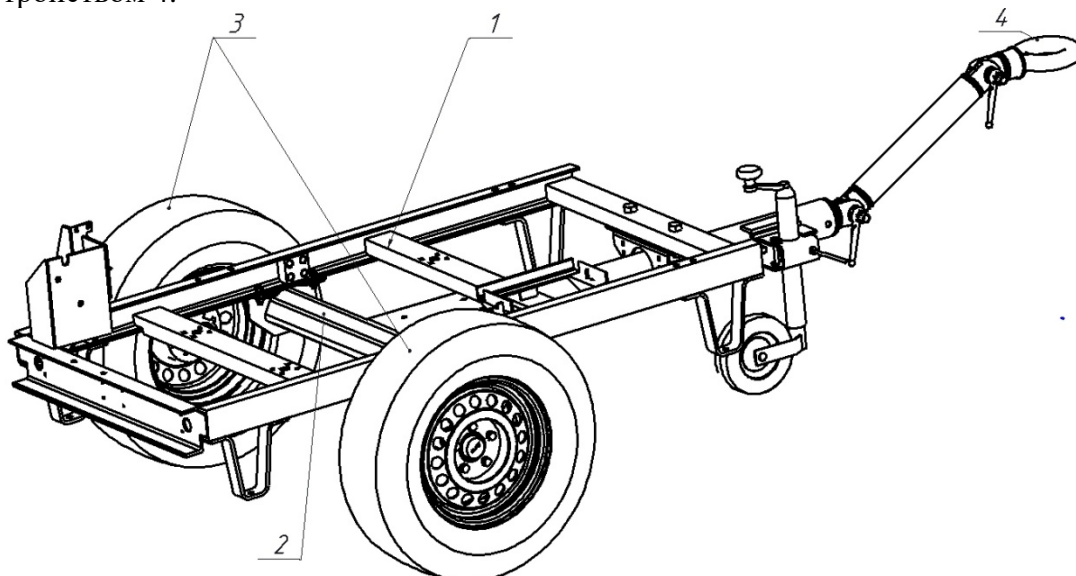
Рисунок 6 – ходовая часть
