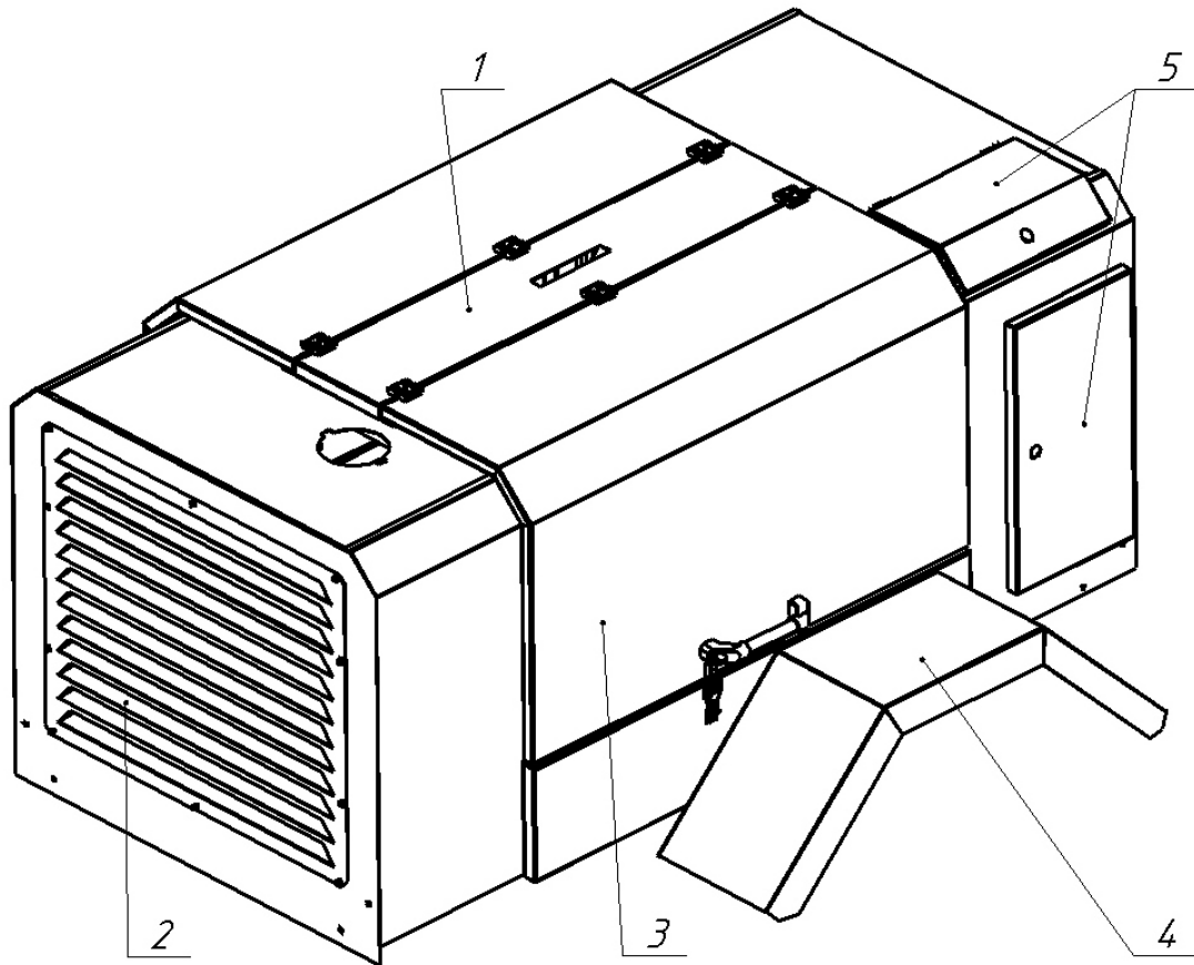
Рисунок 7 - кожух
