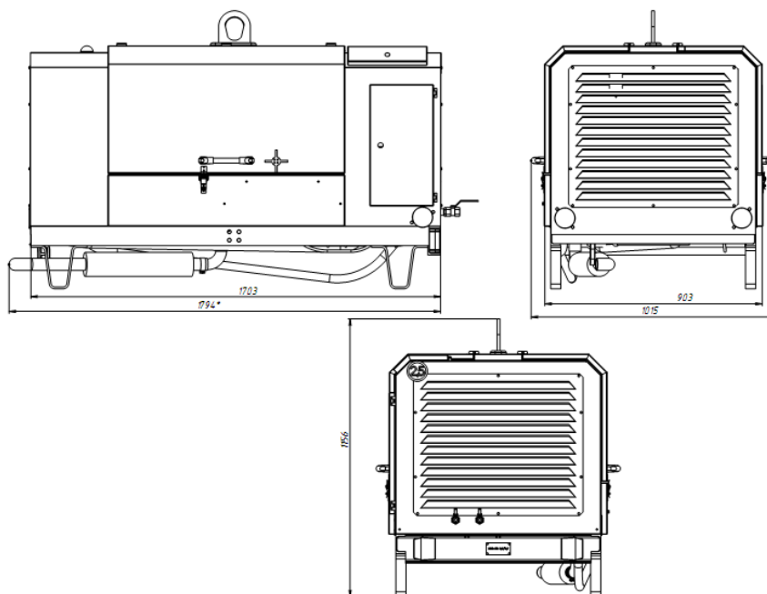
Рисунок 1б исполнение без шасси ММЗ-ПВ3,5/0,7А( б/ш)
