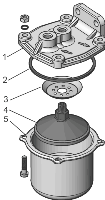
Рисунок 26 - Промывка фильтра грубой очистки топлива
