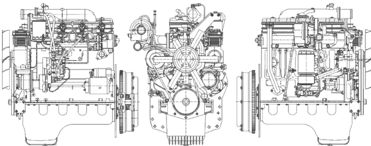
Рисунок 1 – Общий вид дизеля Д–245.7
