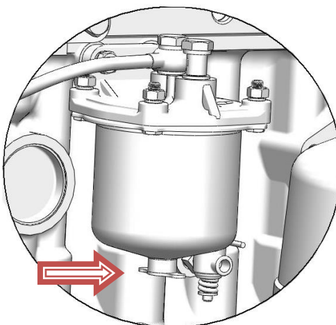
Рисунок 16 - Слив отстоя из фильтра тонкой очистки топлива
