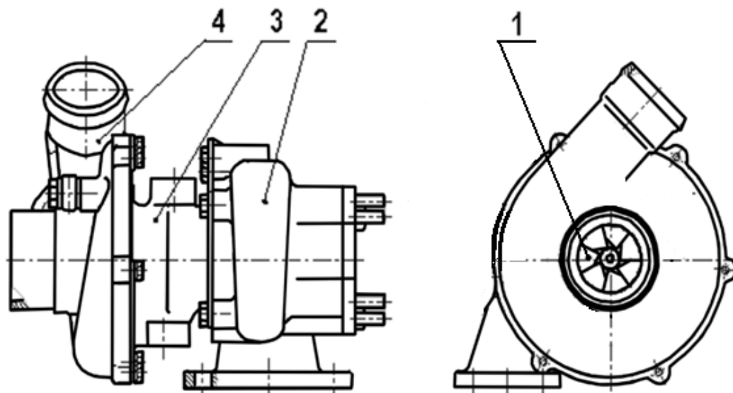
Рисунок 14 – Турбокомпрессор нерегулируемый для дизеля Д-245.12С
