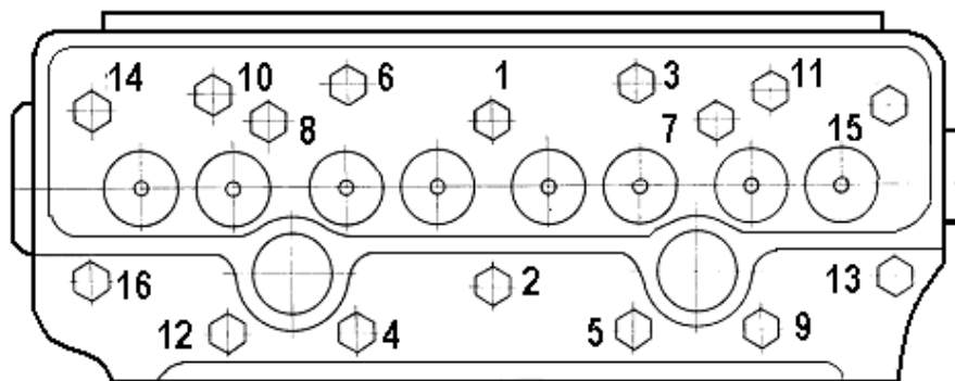
Рисунок 33 - Схема последовательности затяжки болтов крепления головки цилиндров
