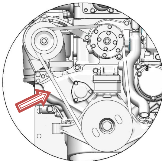
Рисунок 17 - Проверка натяжения ремня вентилятора.
