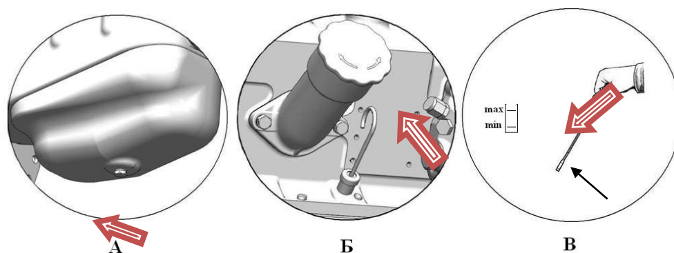
Рисунок 19 – Порядок замены масла в картере дизеля
