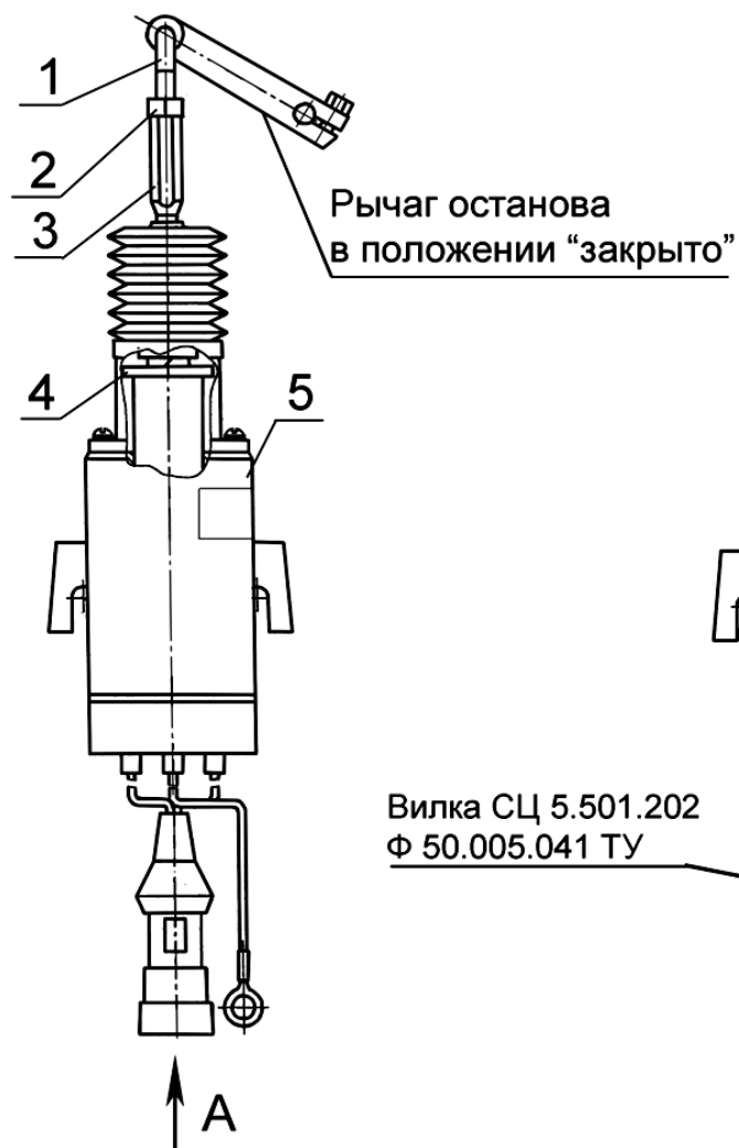
Рисунок 8 – Схема установки электромагнита останова
