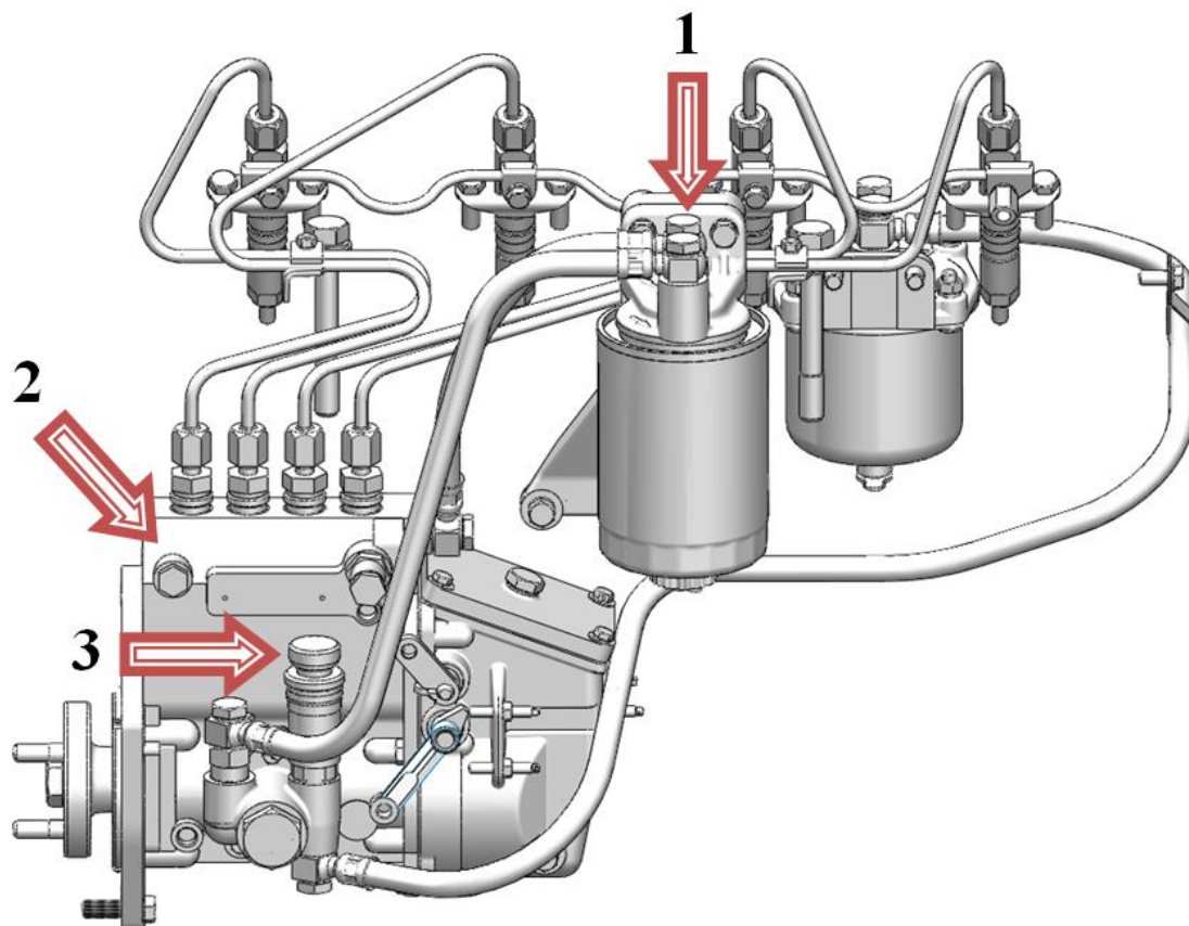
Рисунок 25 – Схема прокачки топливной системы
