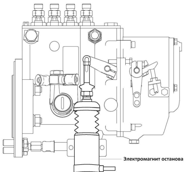
Рисунок 7 – Топливный насос высокого давления РР4М10Р1f с электромагнитом останова (фирмы «Моторпал», Чехия)
