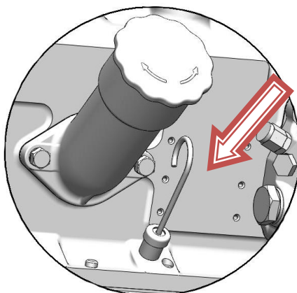
Рисунок 15 - Проверка уровня масла в картере дизеля
