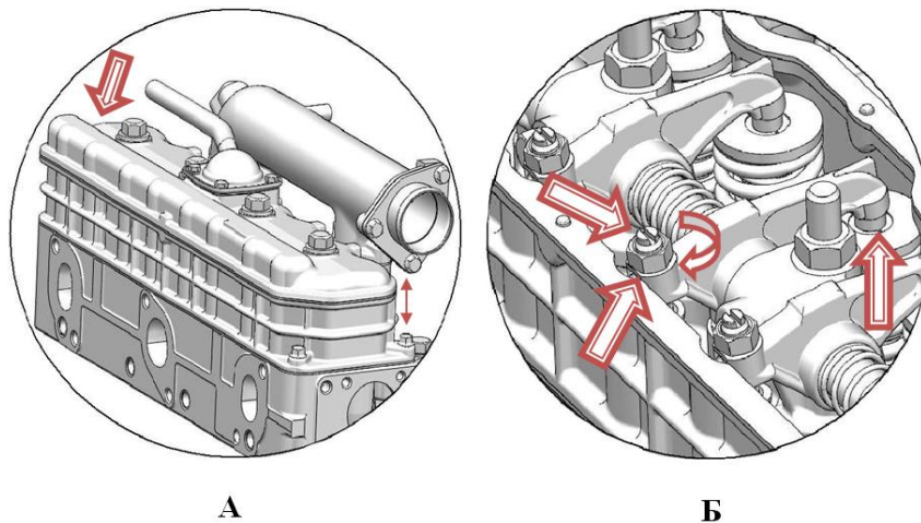
Рисунок 22 - Регулировка зазора в клапанах
