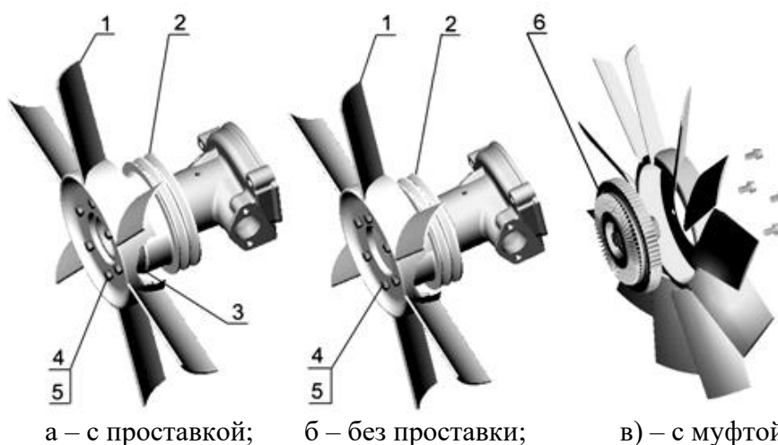
Рисунок 10 – Установка вентилятора
