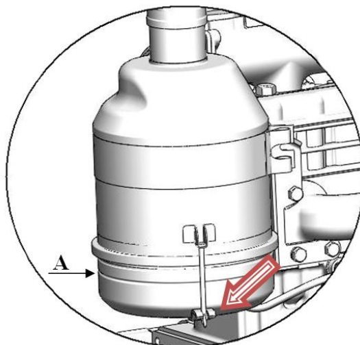
Рисунок 18 – Проверка уровня масла в поддоне воздухоочистителя.
