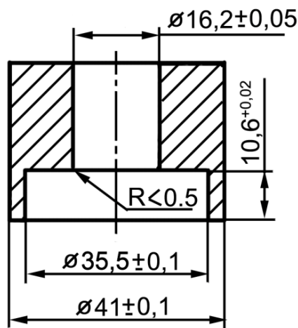
Рисунок 35 - Оправка для запрессовки уплотнения водяного насоса
